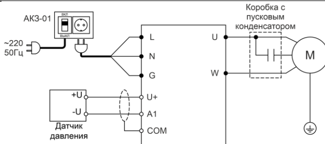
Рисунок 4 – Схема подключения ПЧ
