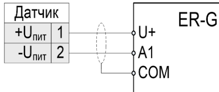
Рисунок 7 – Схемы подключения датчика давления АДМ-100 в корпусе IP20 и IP54
