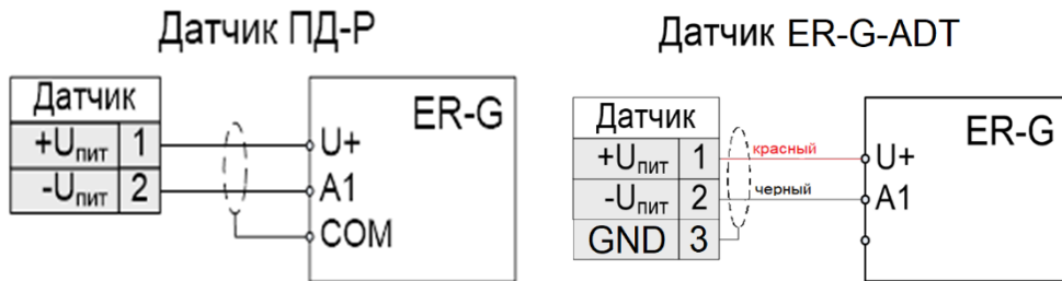
Рисунок 6 – Подключение датчика давления ПД-Р и ER-G-ADT.
