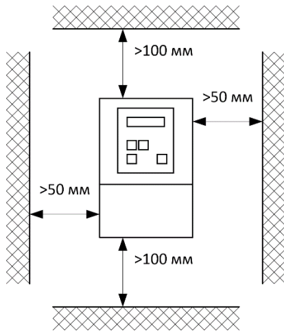
Рисунок 3 – Установка ПЧ
