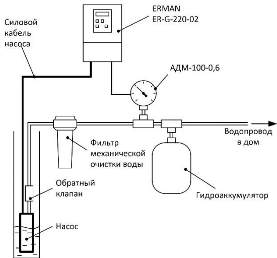
Рисунок 1 – Схема автоматизации системы водоснабжения
